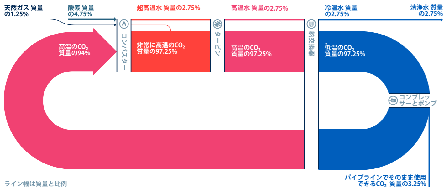
図21 ALLAM-FETVEDTサイクル工程の流れ 情報源: 8 Rivers Capital (提供)
